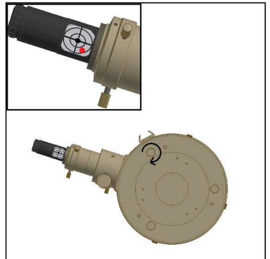
Abb. 4. Den Laser-Kollimator in das Gleitrohr des Okularauszugs einsetzen. Den Kollimator genau wie ein Okular befestigen.
