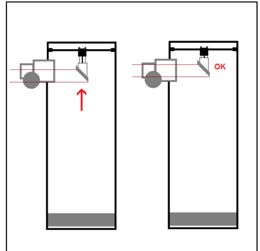
Abb 6. Bewegen Sie den Fangspiegel auf oder ab.
